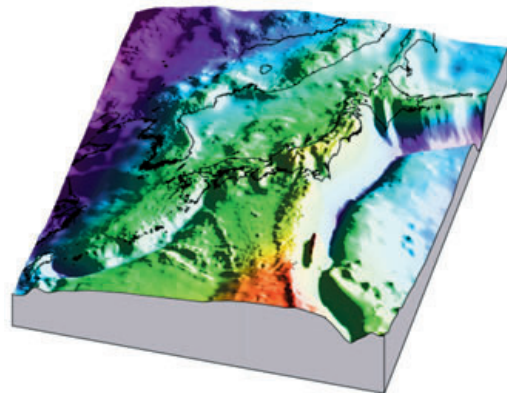
Fig. 5 Relief map of JGEOID2000.
