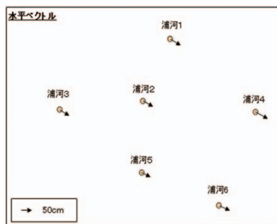
図－3 水平変動ベクトル
