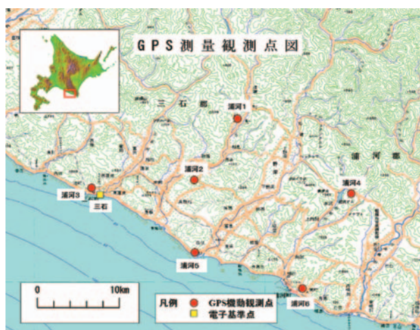
図－2 地殻変動観測点位置図
