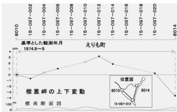
図－7 十勝沖地震に伴う水準点上下変動グラフ
