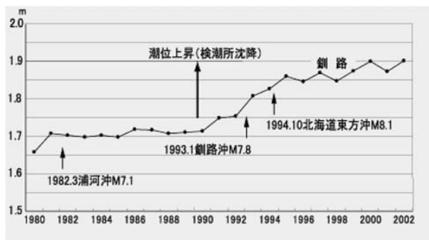
図－8 釧路検潮所の平均潮位グラフ
