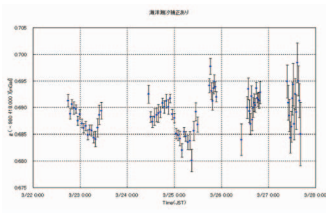
図－15 帯広 FGS における重力値の時間変化 測定期間 2004 年 3 月 22 日～28 日
