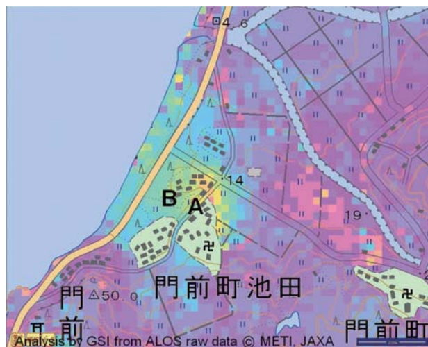
図-11 輪島市門前町池田付近の地殻変動差分画像。A、Bから撮影した写真がそれぞれ写真-3、写真-4である。
