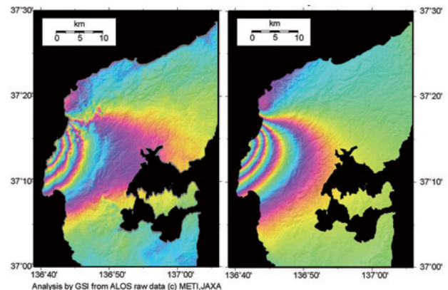
図－1 SAR 干渉画像
