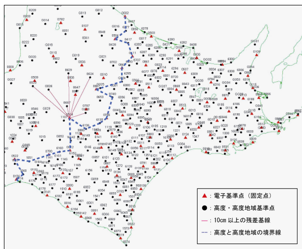
図－3 三次元網平均による基線ベクトル残差評価図
