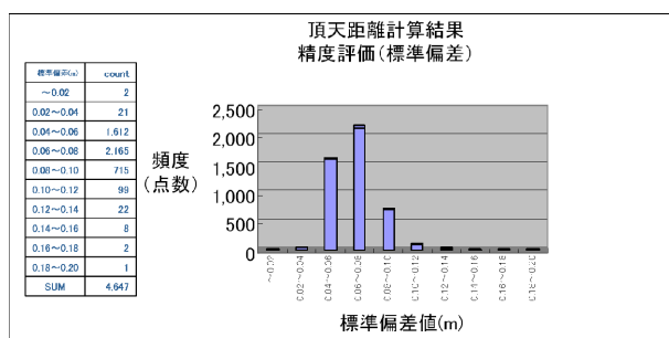
図－5 高低同時網平均計算の標準偏差グラフ
