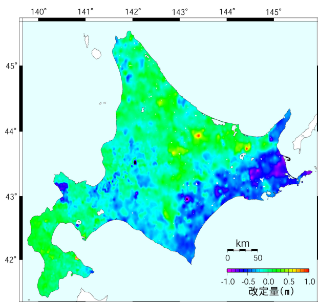
図-8 標高補正パラメータ構築に用いた三角点の標高改定量(4,897点)
