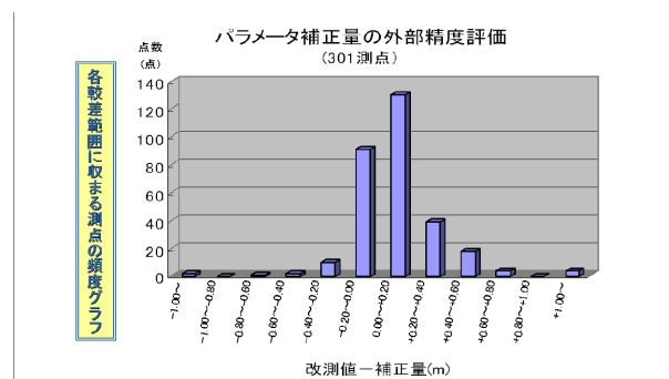
図-9 標高補正パラメータの外部精度評価結果
