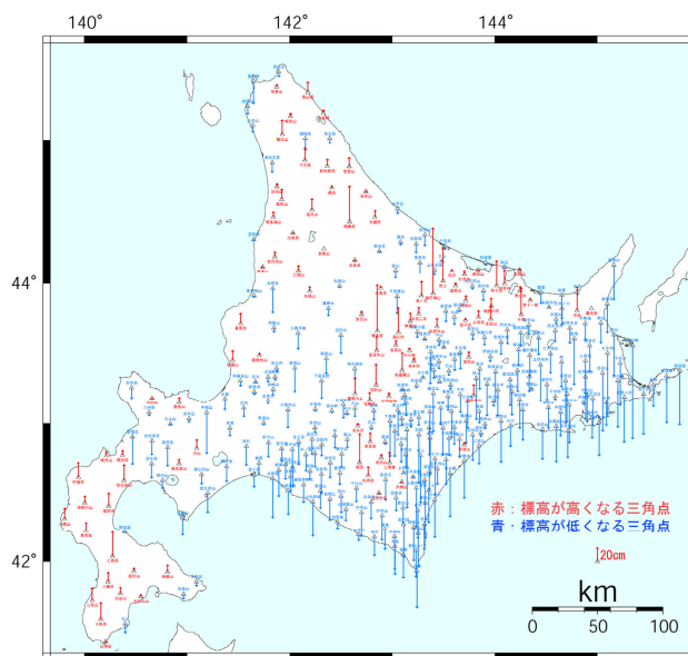
図－4 高度地域基準点の標高改定量図
