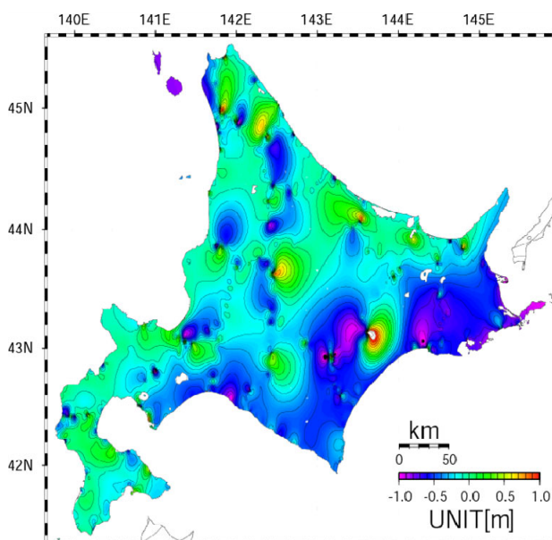
図－1 水準点から求めた約 100 年間の標高変動量
