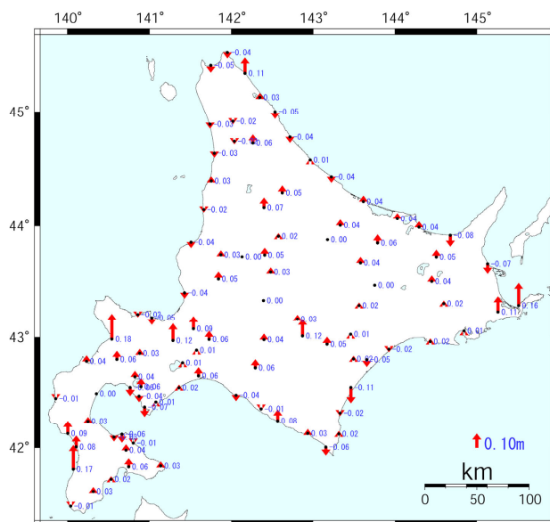
図-2 付属標標高値と測標水準値との較差
