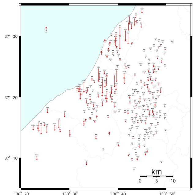
図－14 標高補正パラメータ構築に用いた変動データ
