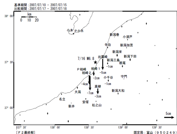
図-2 電子基準点上下変動ベクトル図
