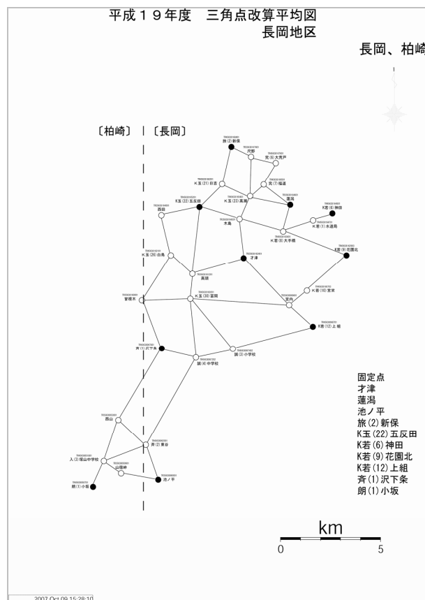
図－8 長岡地区三角点改算平均図
