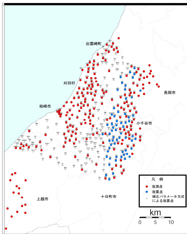
図－12 補正パラメータ方式により改算成果を求める三角点の配置状況図
