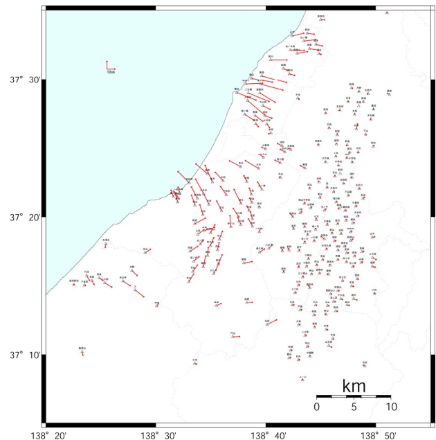
図－13 座標補正パラメータ構築に用いた変動データ
