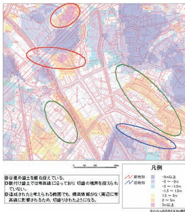
図-9 盛土地形の計測結果（マップデジタイズ法）
