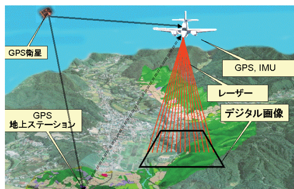
図-2 航空レーザ測量イメージ図
