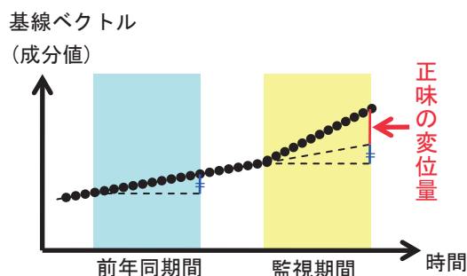
図－2 基線ベクトル変位量成分値の差（初期版）
