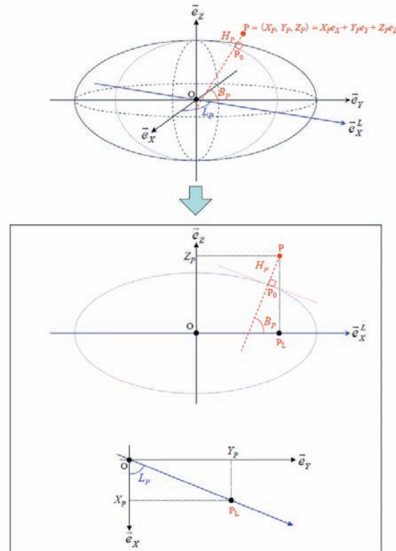
図-8 測地座標
