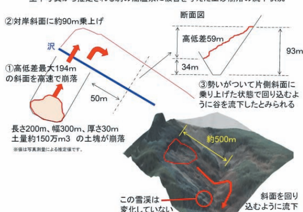
図-2 平成20年岩手・宮城内陸地震の際に作成した写真図の一部(上図)と解析結果の一部(下図)
