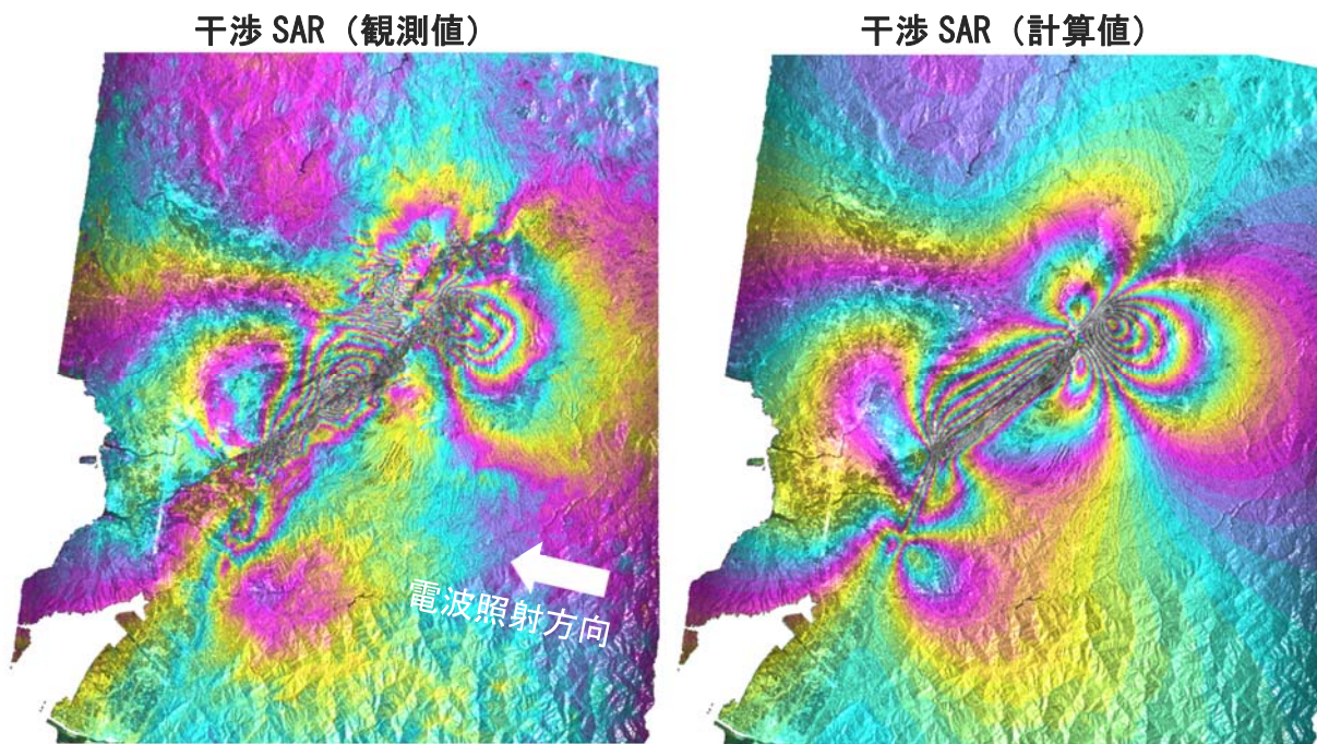
図2 (左) 干渉 SAR 画像. 1 回目観測 : 2016/03/07 2 回目観測 : 2016/04/18 (右) 震源断層モデルから予想される干渉画像
