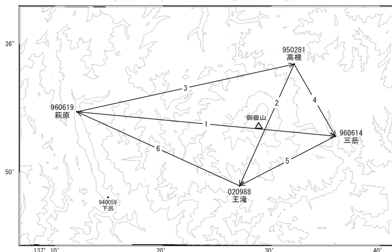
御嶽山周辺 GNSS連続観測基線図
