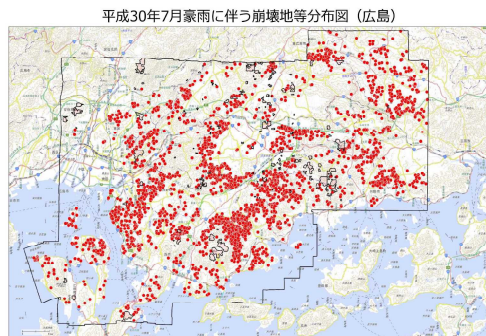
平成30年7月豪雨に伴う崩壊地等分布図(広島) 写真等資料番号②
