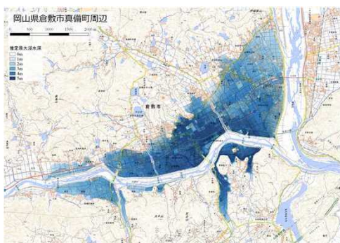
平成30年7月豪雨: 岡山県倉敷市真備町周辺の浸水段彩図 写真等資料番号①
