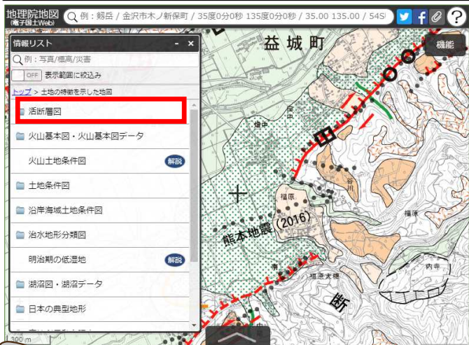
1:25,000活断層図
