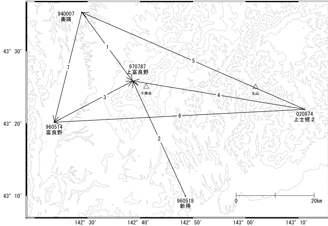
十勝岳周辺 GNSS連続観測基線図
